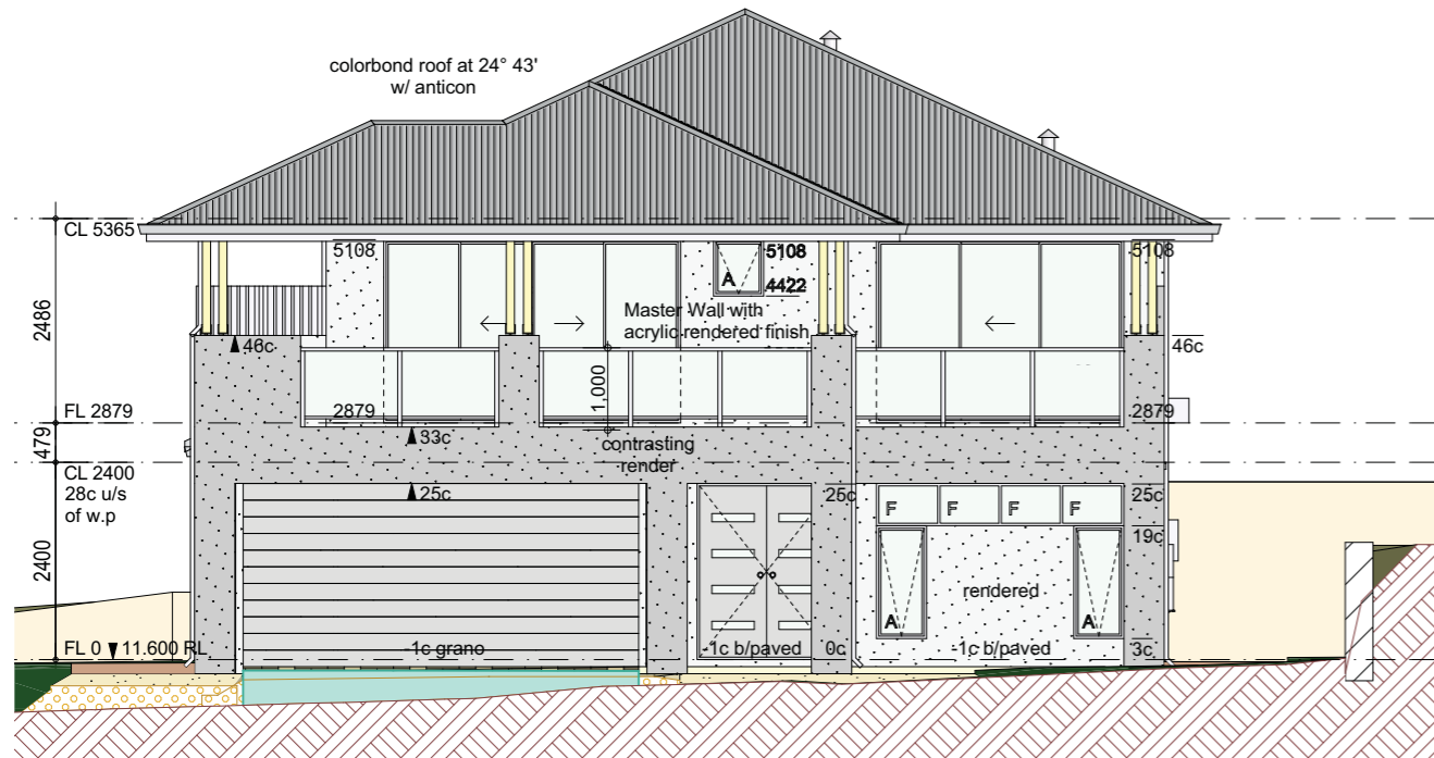
Elevation 1
