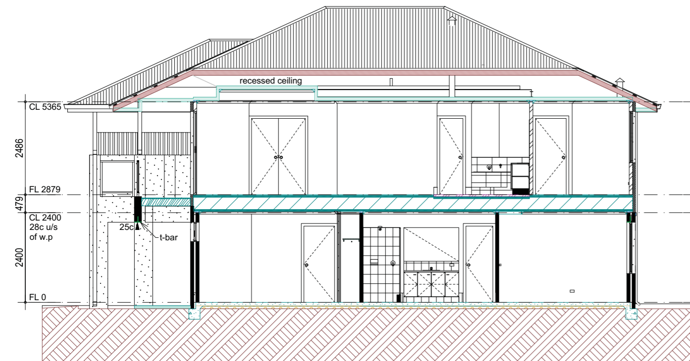
A2 Section
