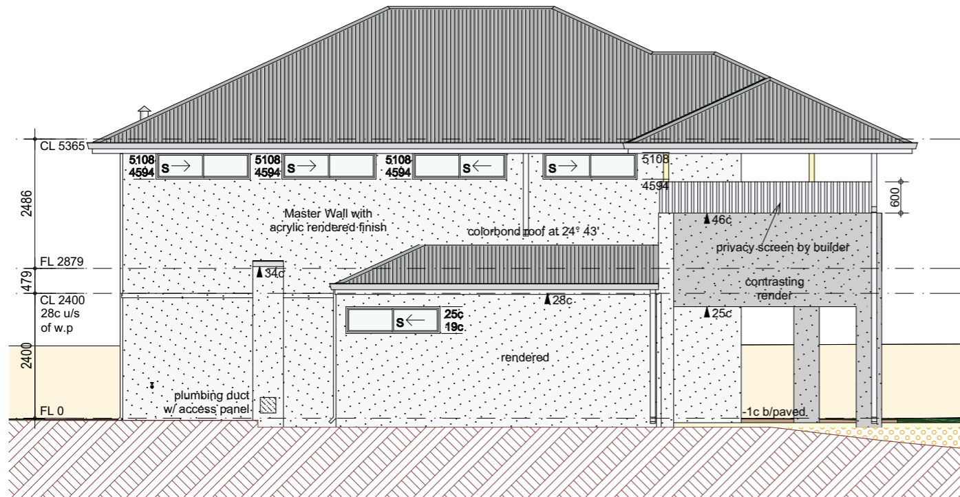
Elevation 4
