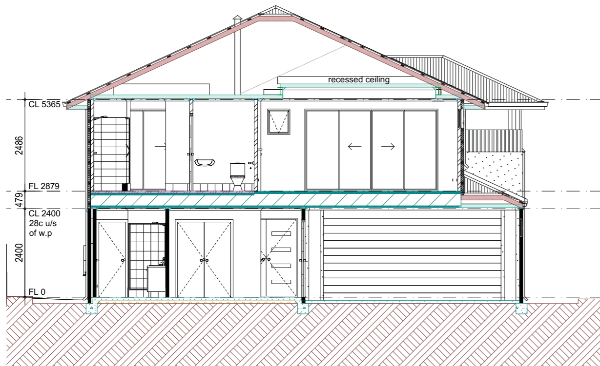
A3 Section
