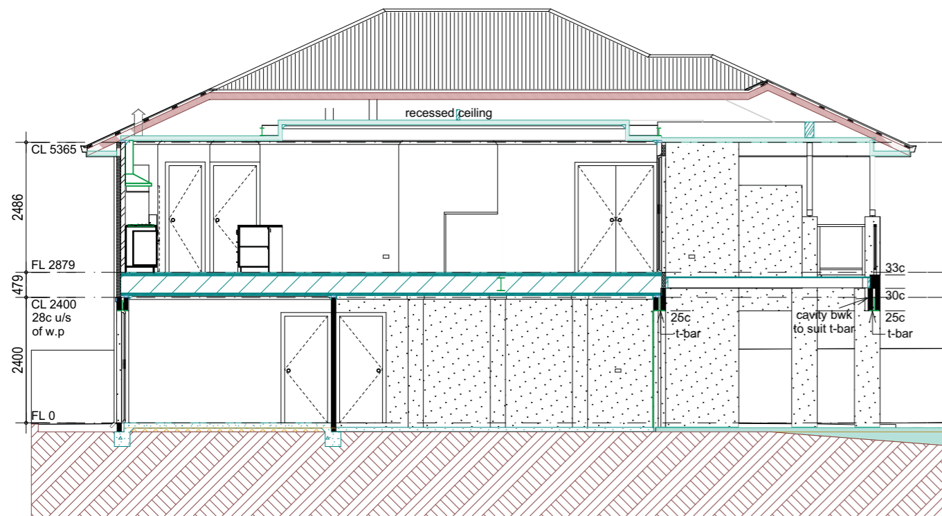
A4 Section
