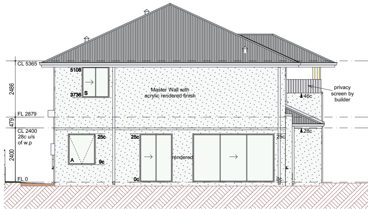
Elevation 3
