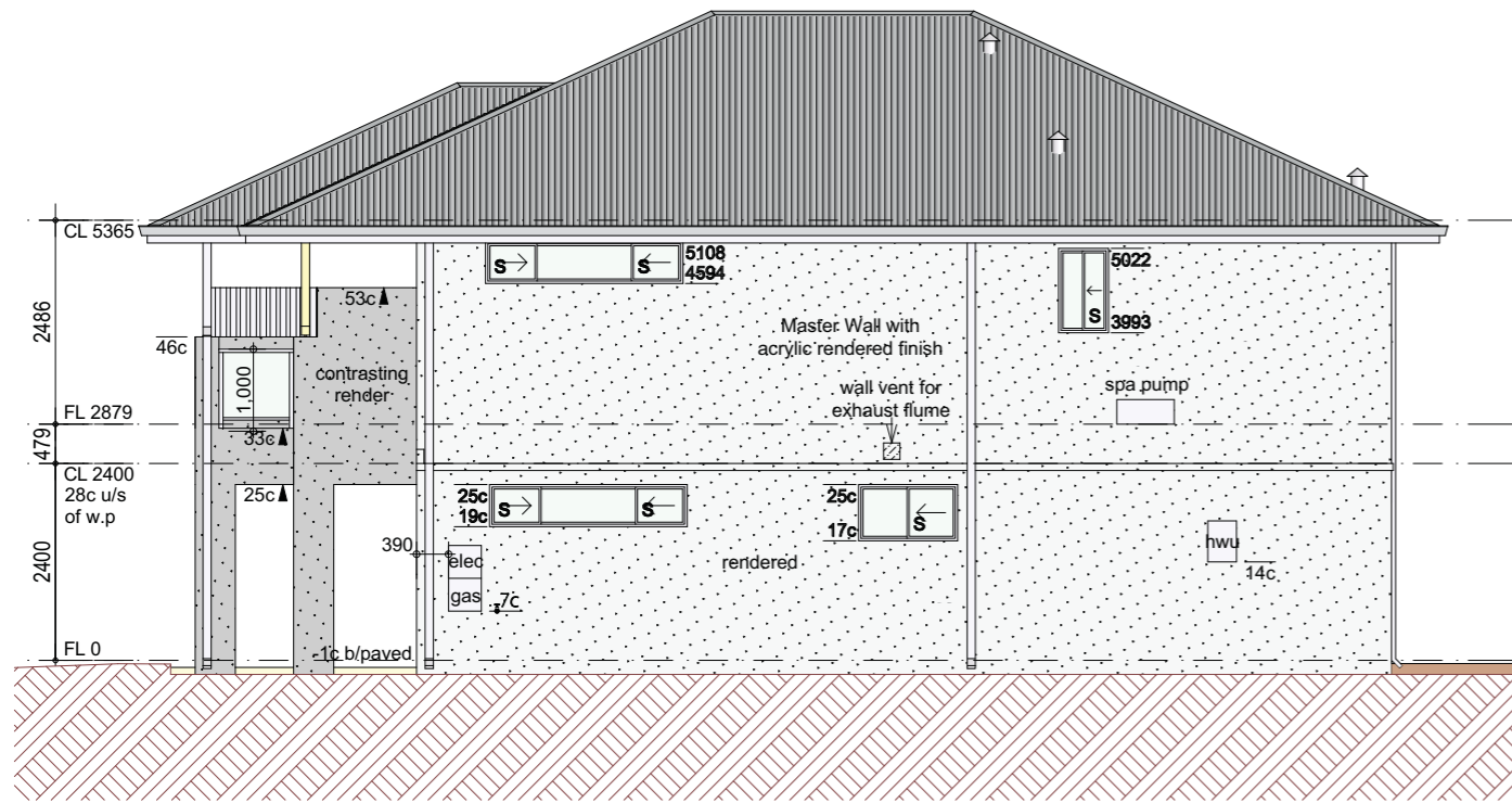
Elevation 2
